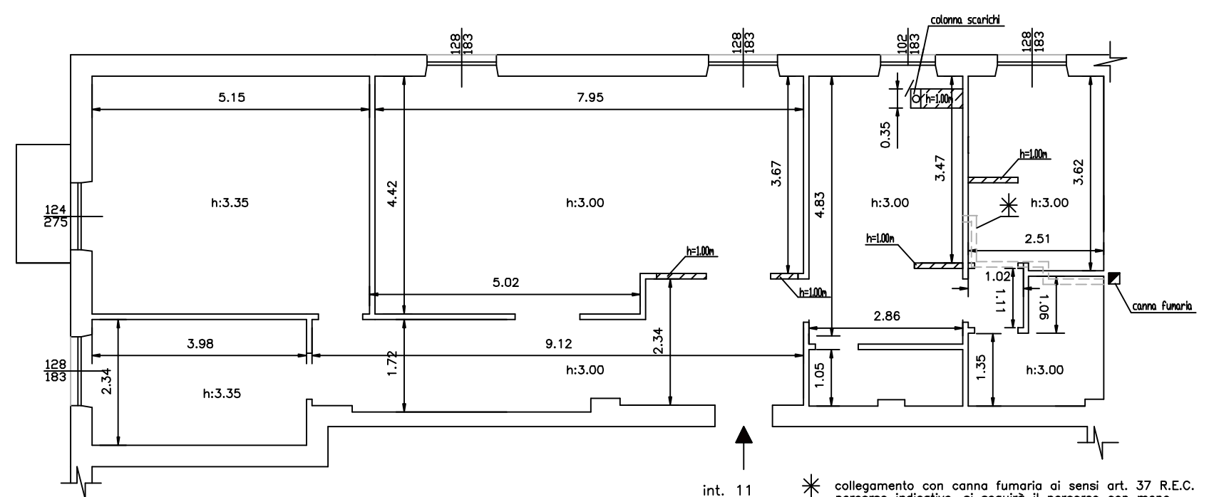
STATO DI PROGETTO
